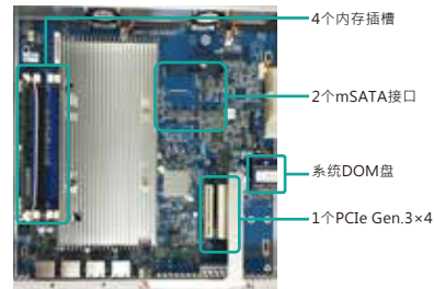
471U 产品主板示意图
