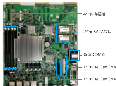
x80U/x80U-SAS 产品主板示意图 注：仅 x80U-SAS 内置 2 个 128GB mSATA 模块
