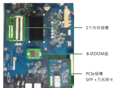
463U 产品主板示意图
