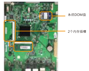
453U 产品主板示意图
