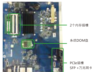
1263U/863U 产品主板示意图
