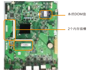
1253U/853U 产品主板示意图
