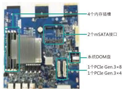
1271U/871U 产品主板示意图
